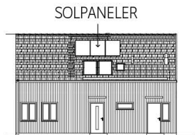
FASAD MOT NORDVÄST
