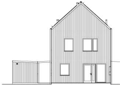
FASAD MOT NORDOST
