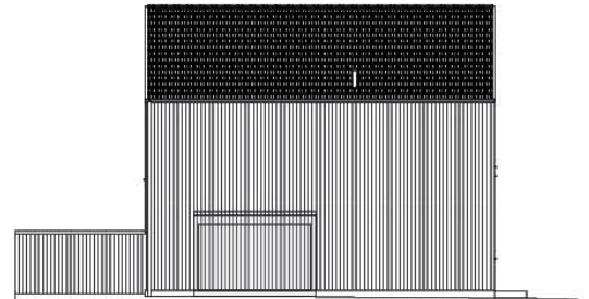
FASAD MOT NORDVÄST
