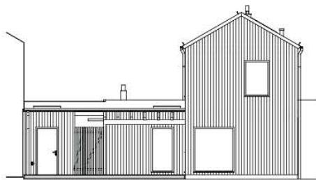
FASAD MOT NORVÄST
