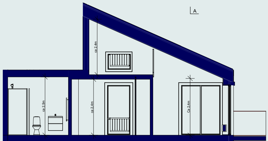
Snitt A-A
