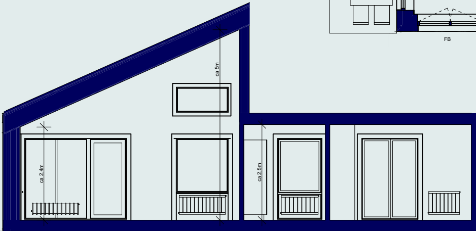
Snitt A-A
