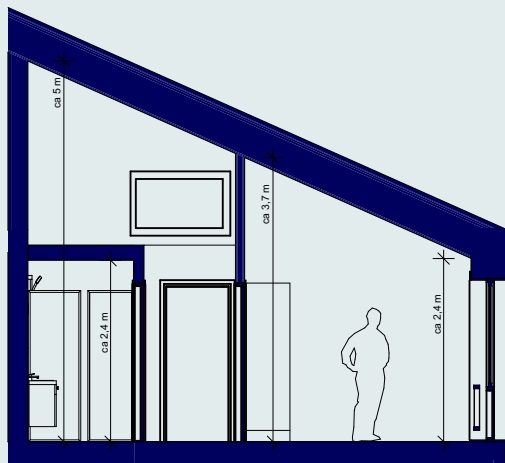
Snitt a-a
