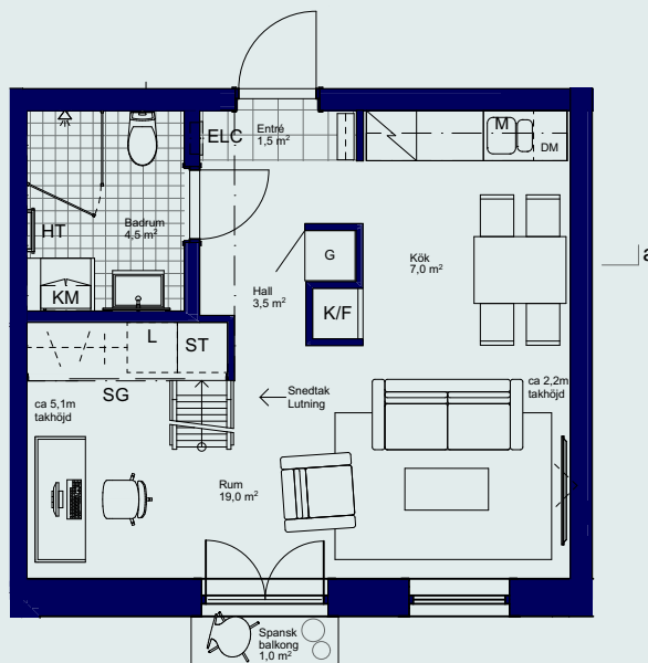
Planlösning
