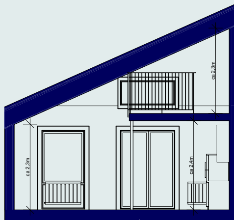
Snitt a-a
