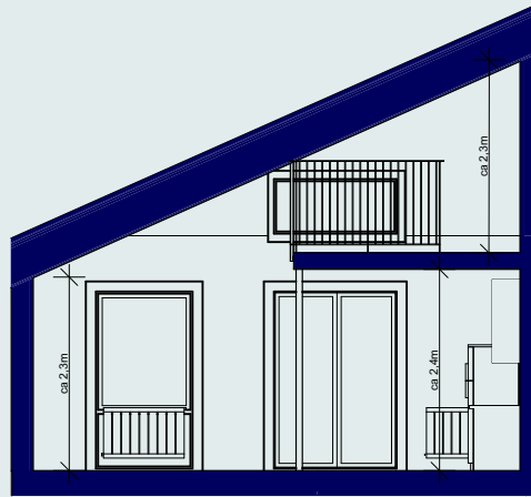
Snitt a-a
