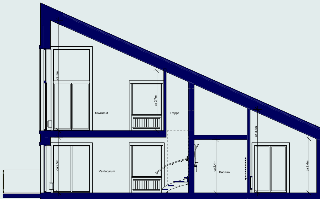
Snitt a-a
