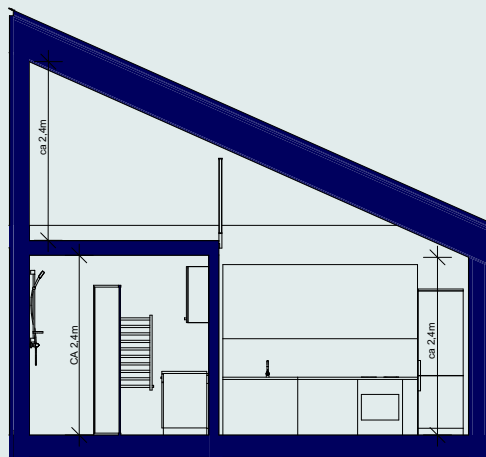
Snitt A-A
