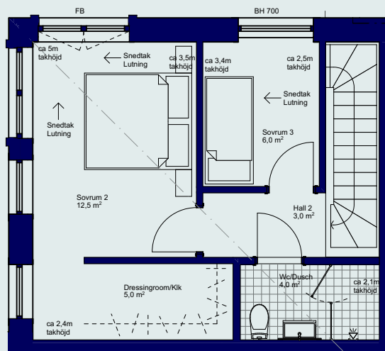
Planlösning övervåning
