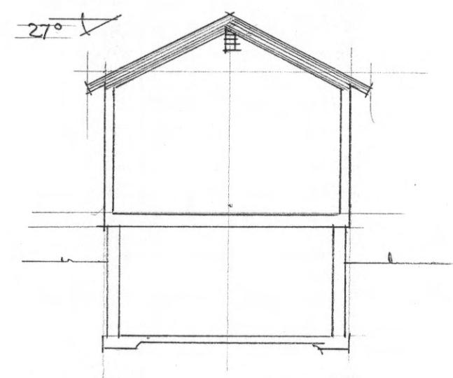
SEKTION A
