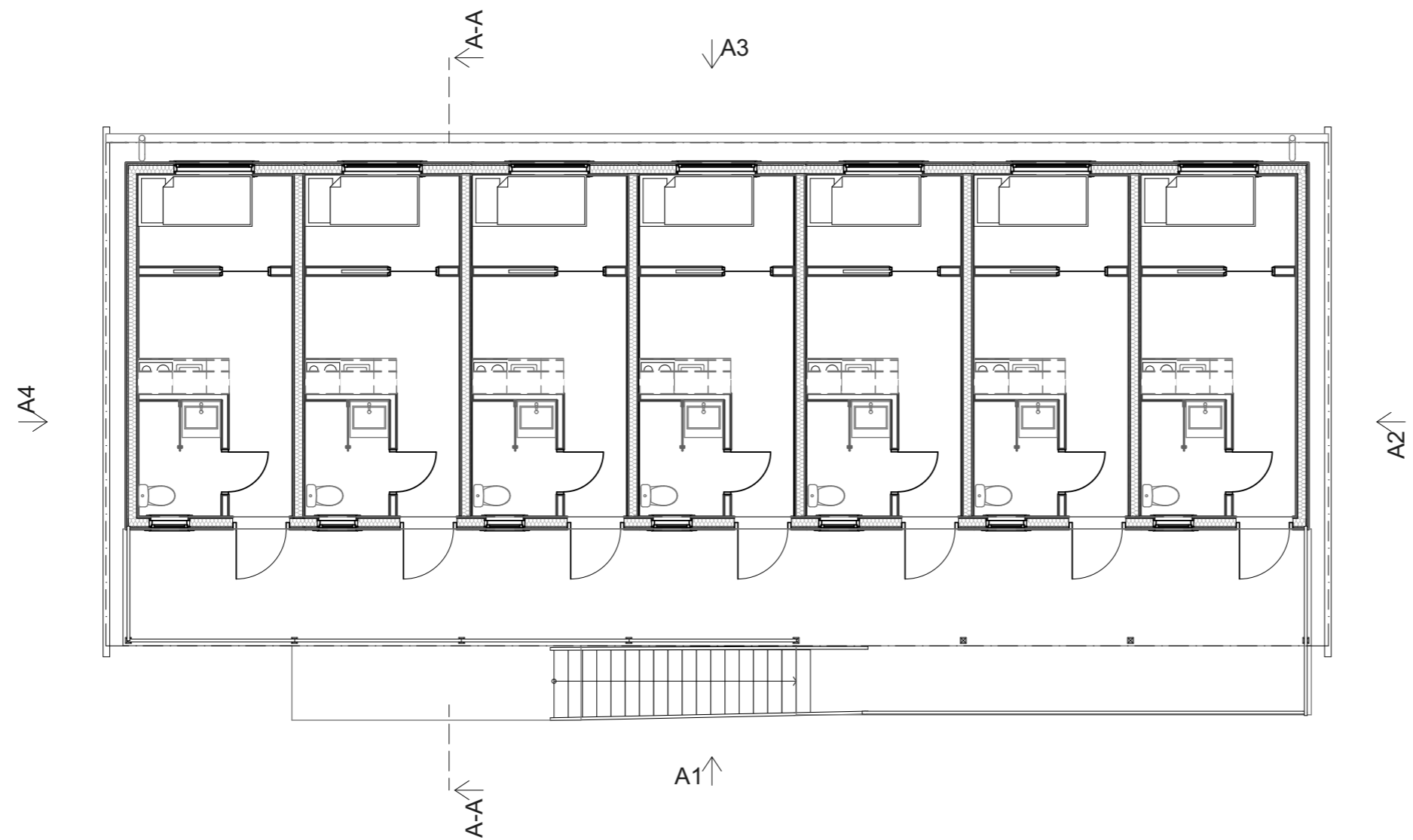
PLAN - ÖVERVÅNING 1:100
