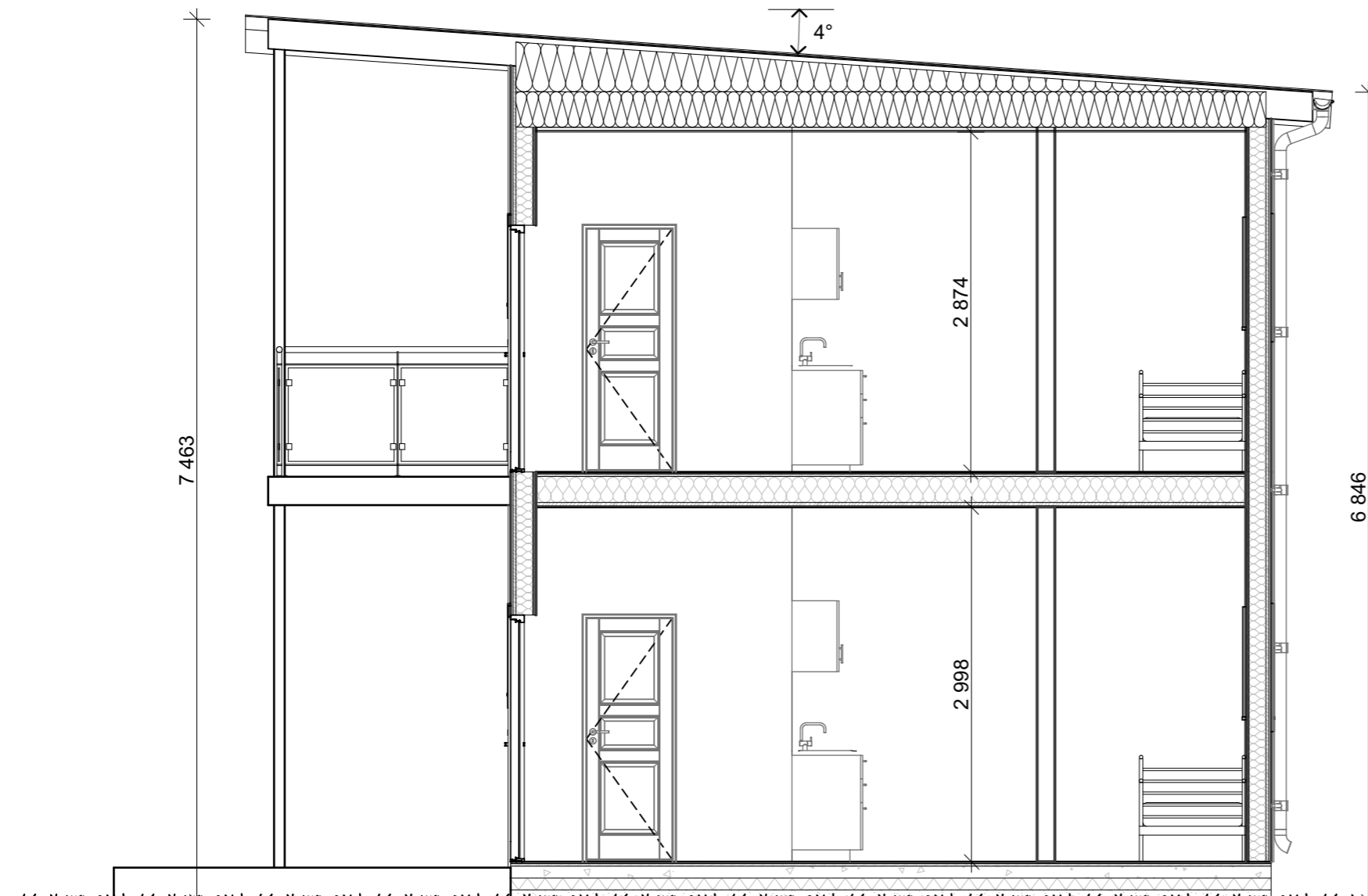
SEKTION A 1:50
