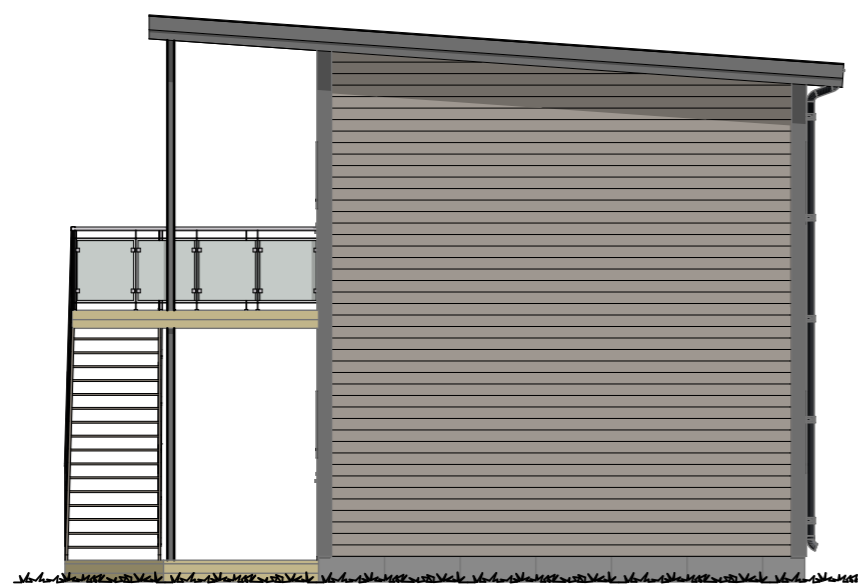
FASAD A2 1:100
