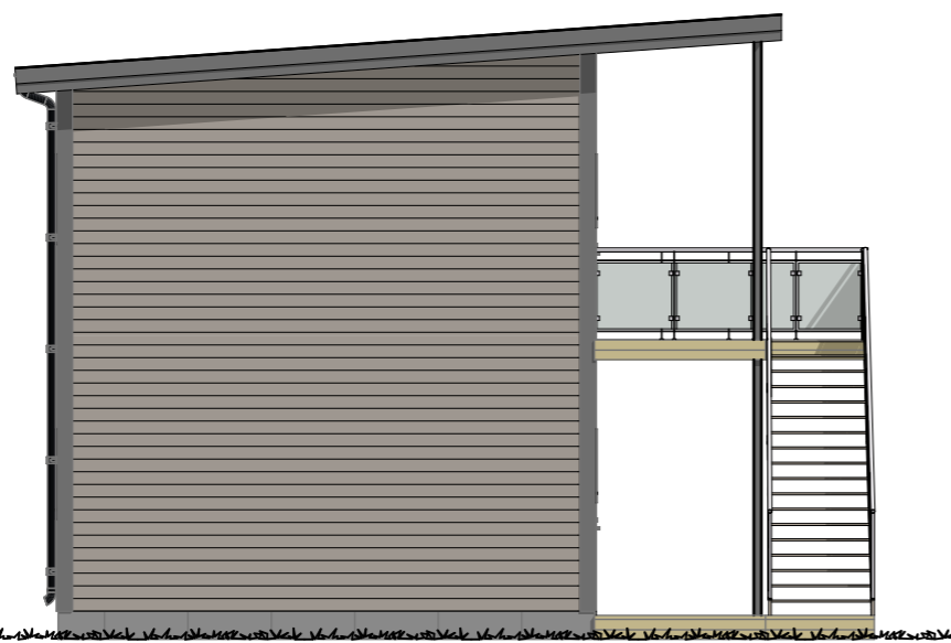
FASAD A4 1:100
