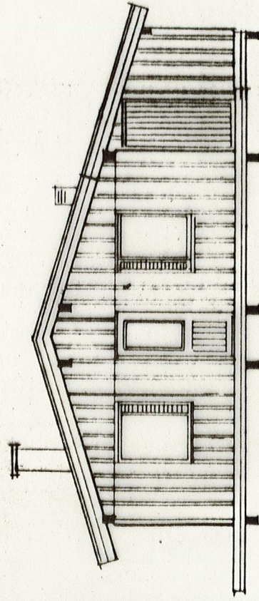
GAVEL SÖDER
