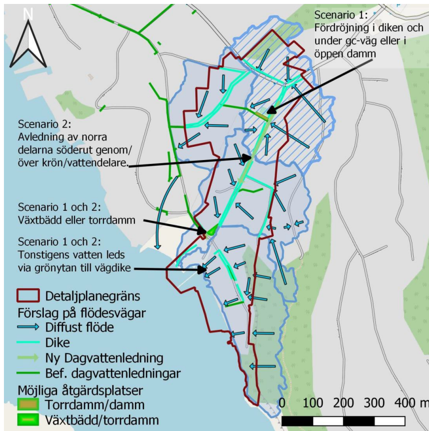
Systemskiss över dagvattenhanteringen med föreslagna avrinningsvägar, fördröjningsmagasin och reningsanläggningar. Åtgärder planeras enligt scenario 1 (WRS 2020).
