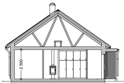
Sektion B (skala 1:200)
