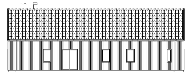
Trädgårdsfasad (skala 1:200)
