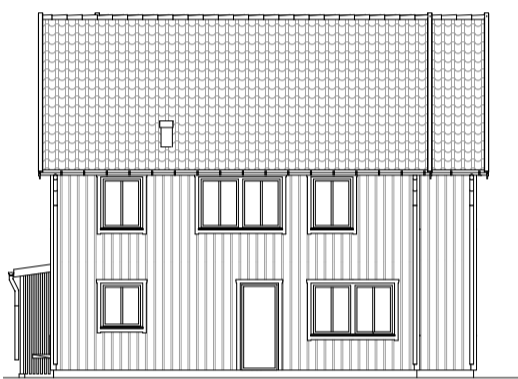
Fasad 4 (skala 1:200)
