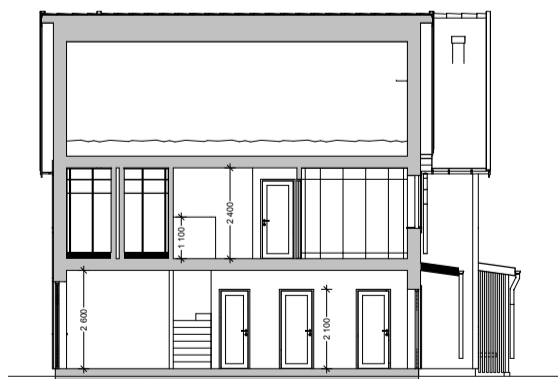
Sektion C (skala 1:200)
