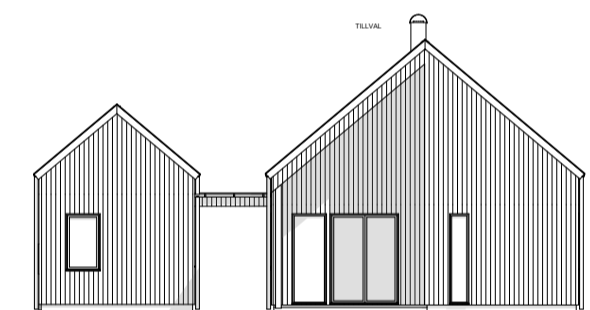
Gavelfasad (skala 1:200)
