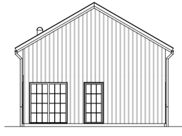
Fasad 4 (skala 1:200)
