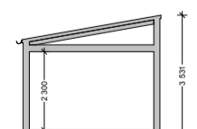
Sektion E (skala 1:200)
