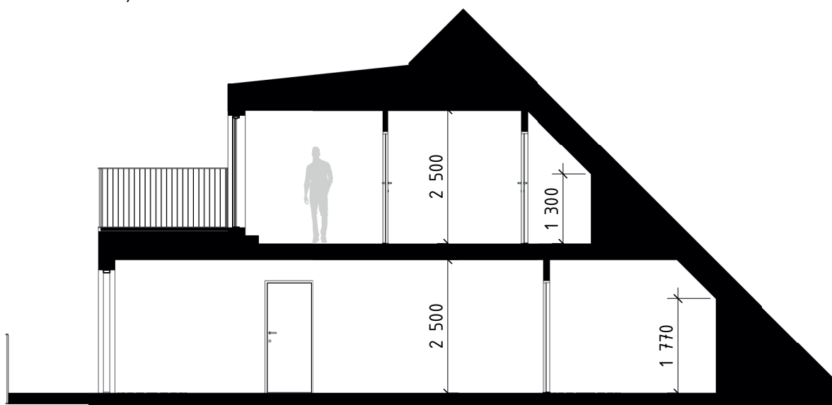
SEKTION B-B (TAKKUPA)
