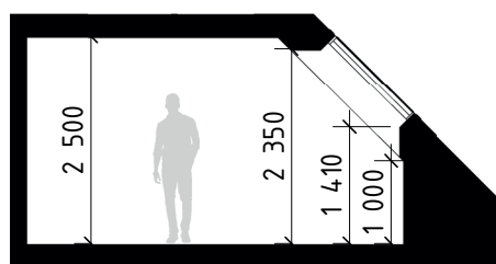
SEKTION A-A (TAKFÖNSTER)
