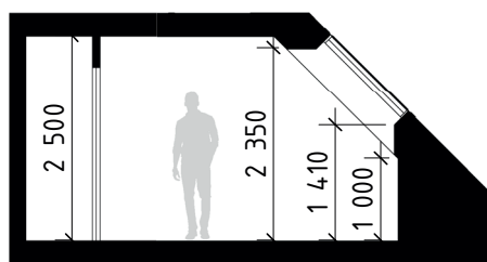
SEKTION A-A (TAKFÖNSTER)
