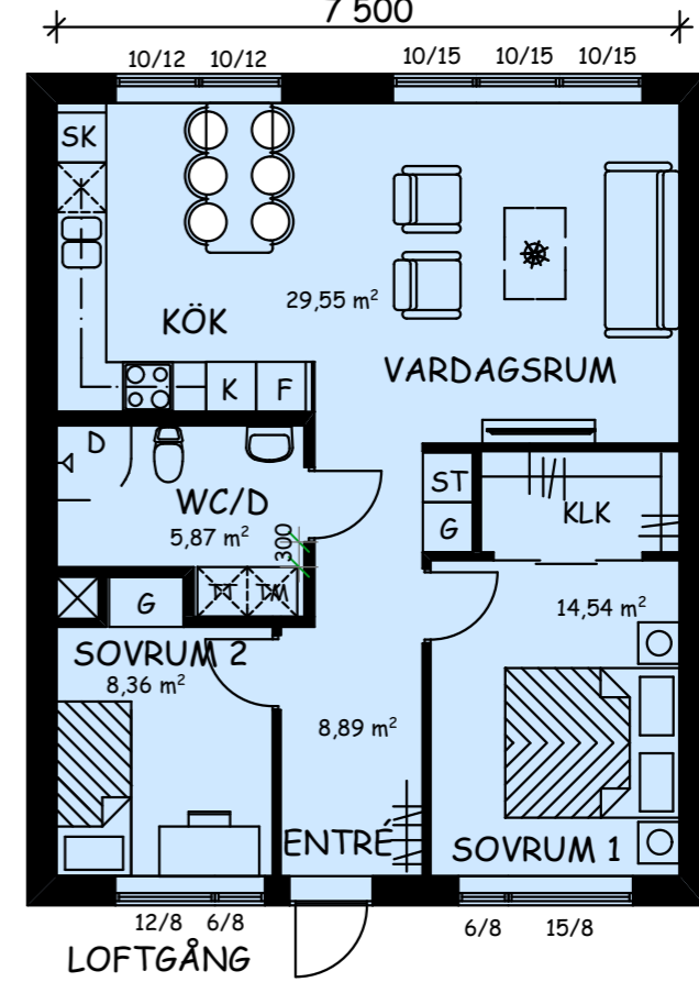
3 ROK Boyta: 70,0 m 2
