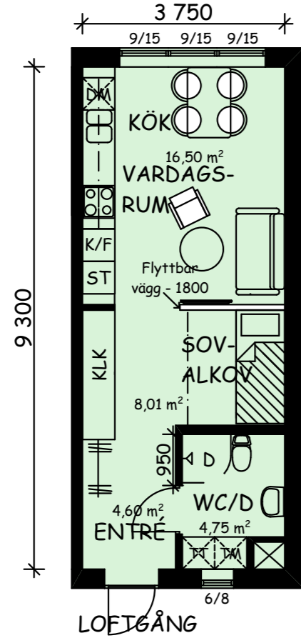
1 ROK med SOVALKOV Boyta: 34,9 m 2
