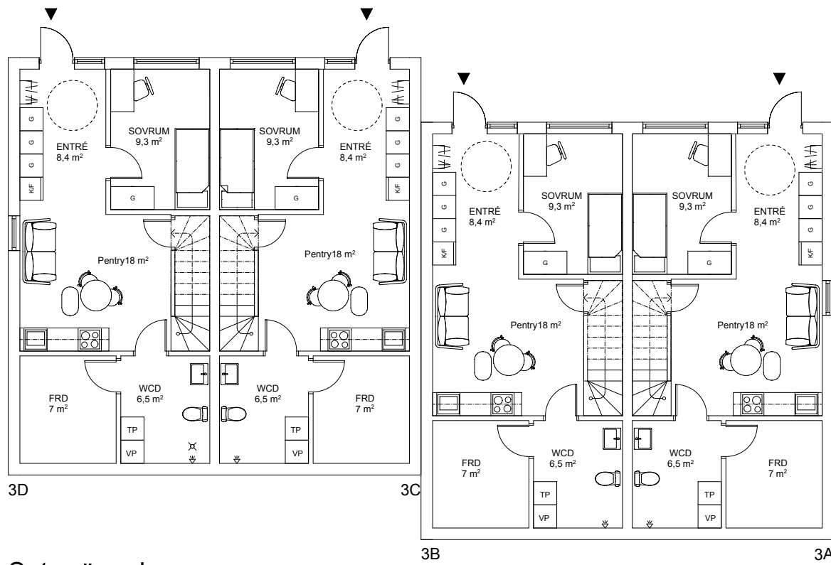
Suterrängplan
