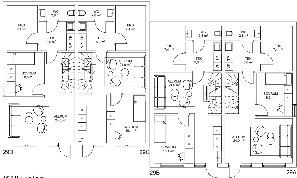
Källarplan
