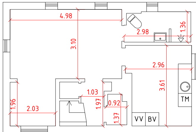
KÄLLARPLAN
