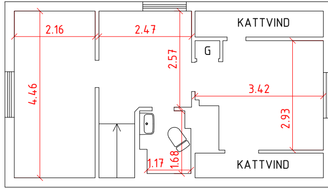
ÖVRE PLAN
