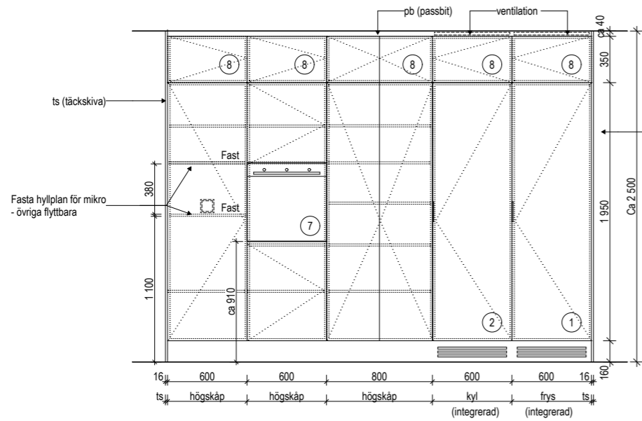
A-A ELEVATION
