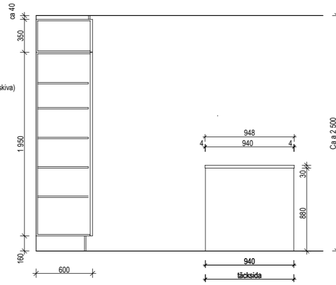
B-B ELEVATION-SEKTION
