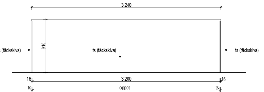
D-D ELEVATION KÖKSÖ
