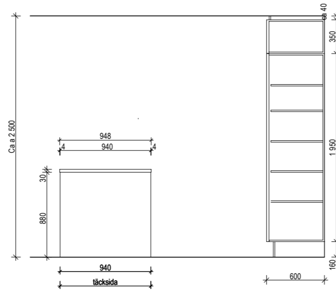
B-B ELEVATION-SEKTION
