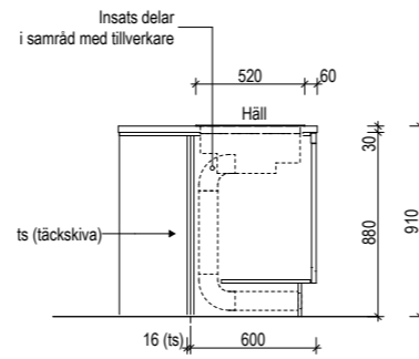
E-E SEKTION GENOM KÖKSÖ
