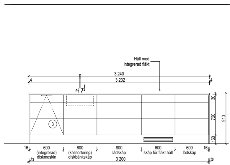
C-C ELEVATION KÖKSÖ MOT KÖK
