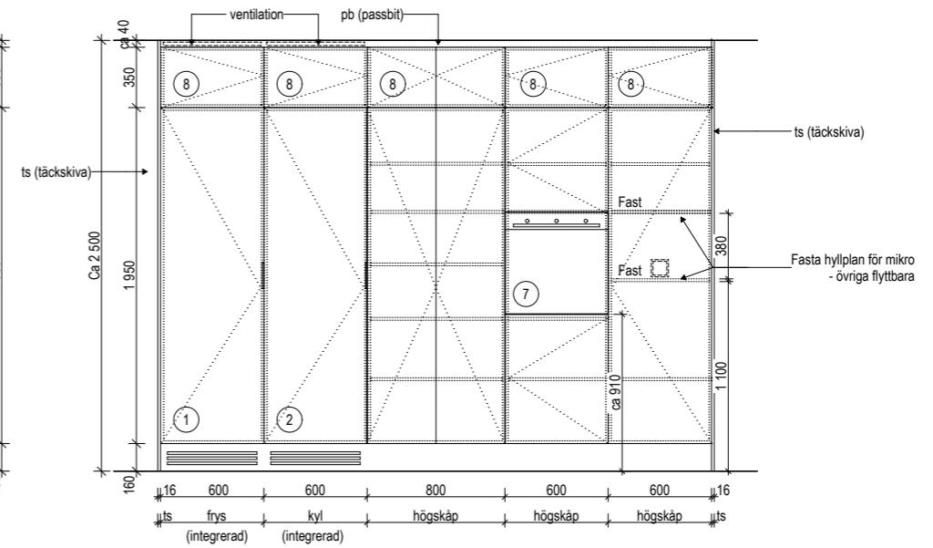
A-A ELEVATION
