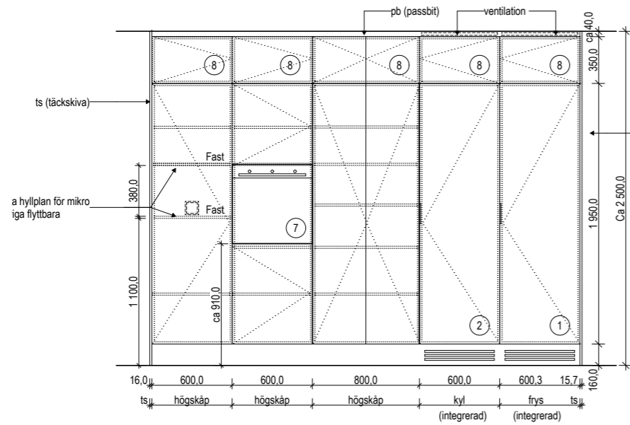
A-A ELEVATION
