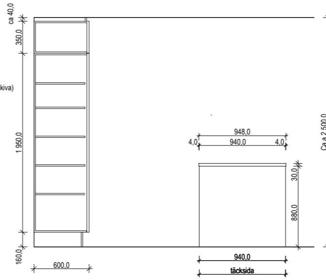
B-B ELEVATION-SEKTION
