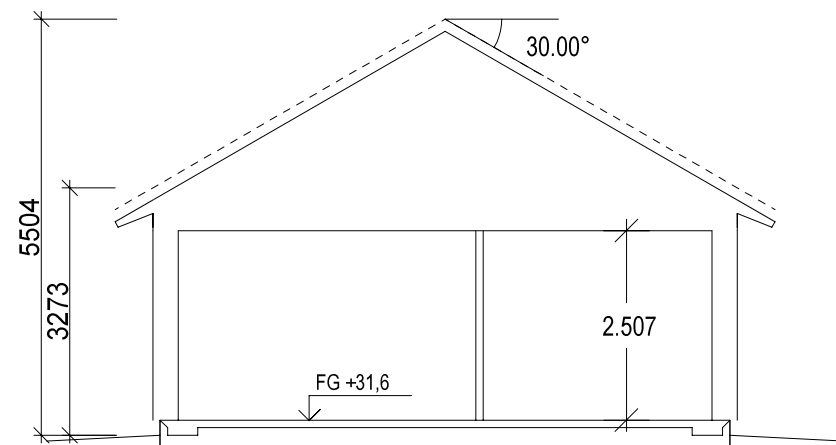
SEKTION A-A
