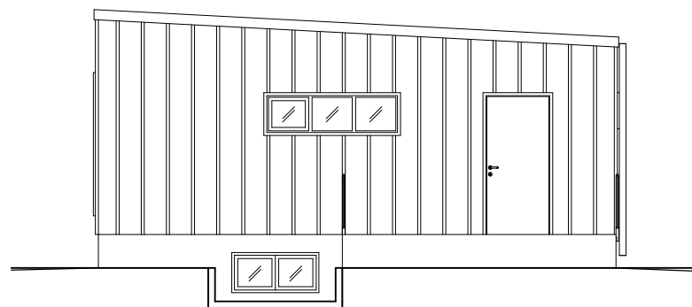
FASAD ÖST
