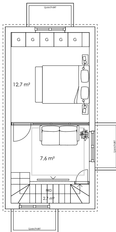
KÄLLARPLAN
