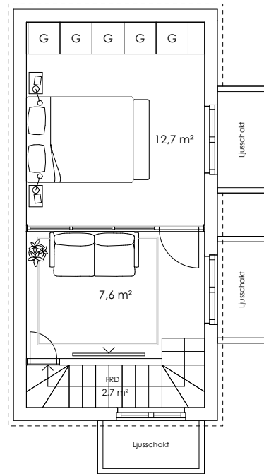
KÄLLARPLAN
