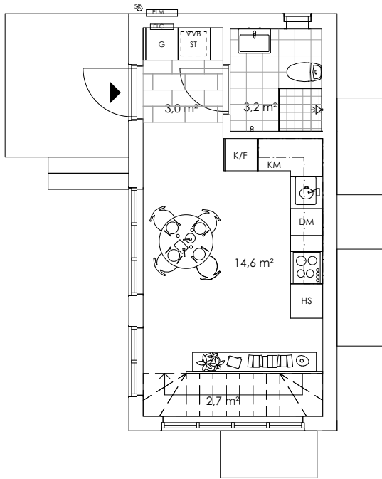
ENTRÉPLAN
