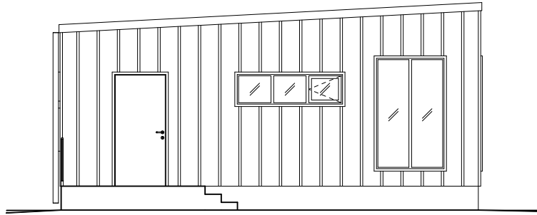
FASAD VÄST
