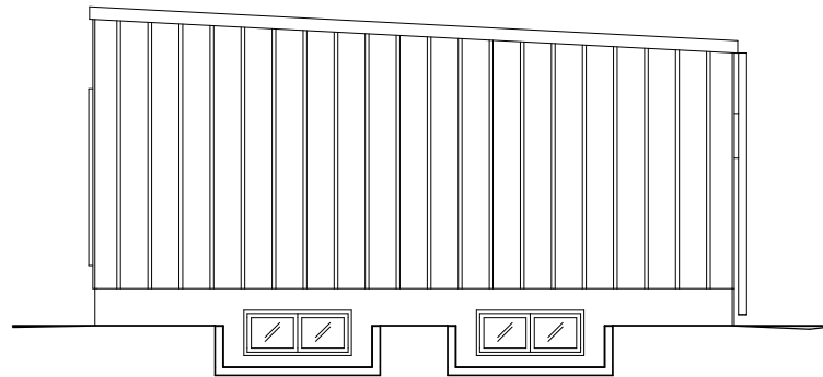
FASAD ÖST
