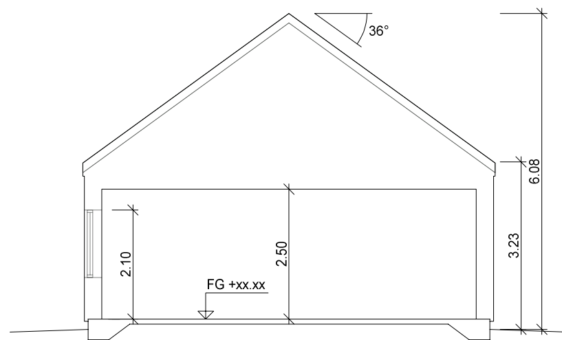
SEKTION A-A
