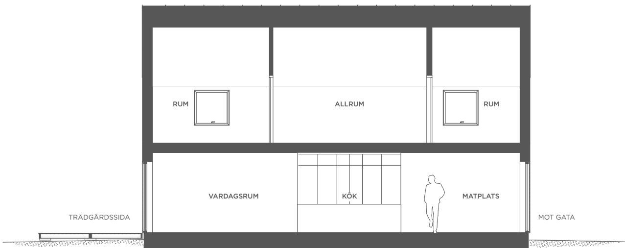
LÄNGDSEKTION CM06
