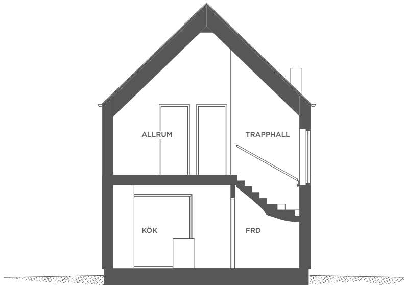
SEKTION CM06
