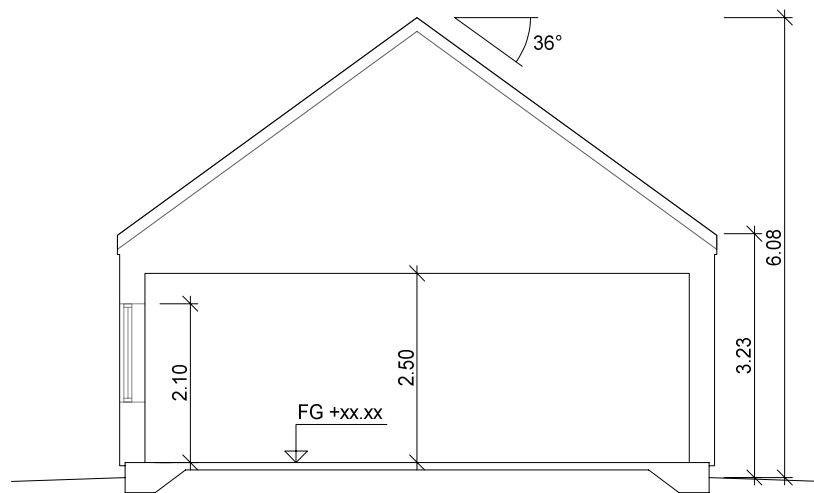
SEKTION A-A
