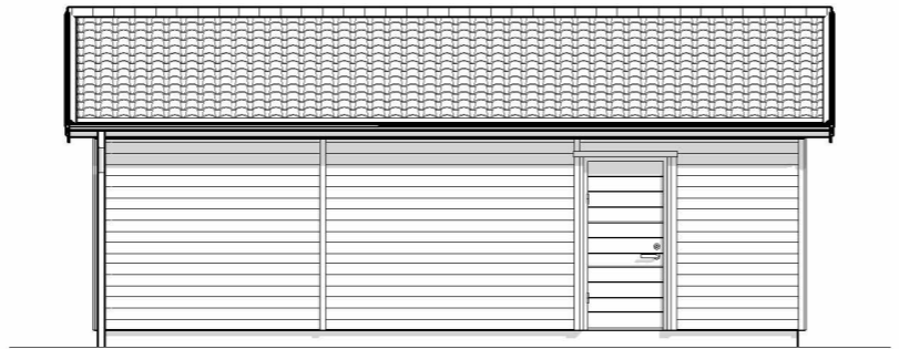
FASAD HÖGERSIDA
