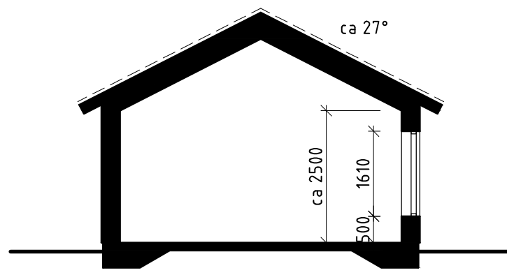
PRINCIPSEKTION B-B
