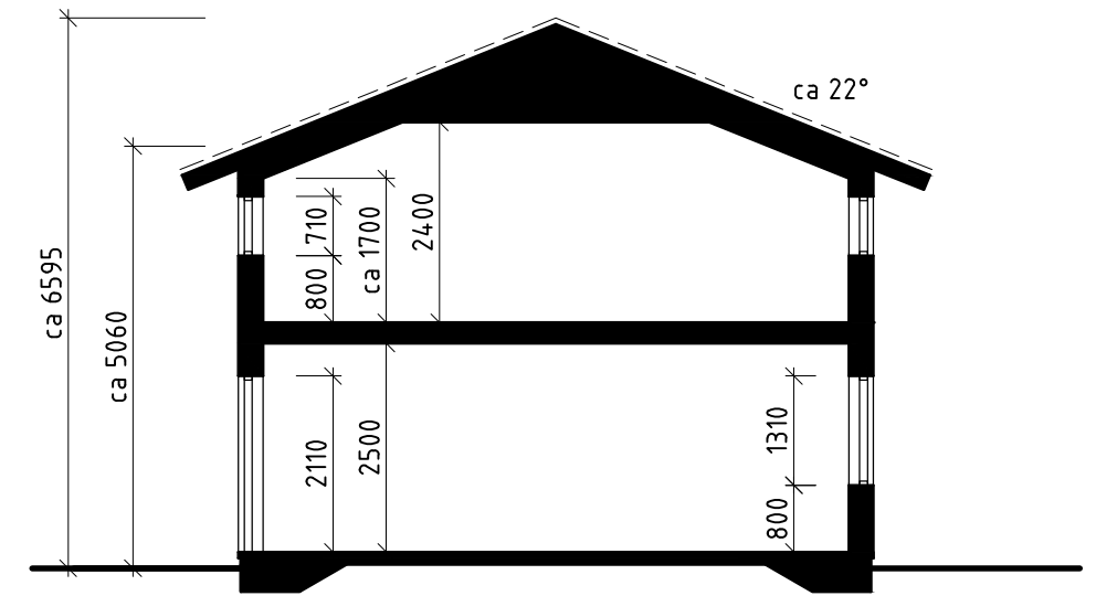
PRINCIPSEKTION A-A
