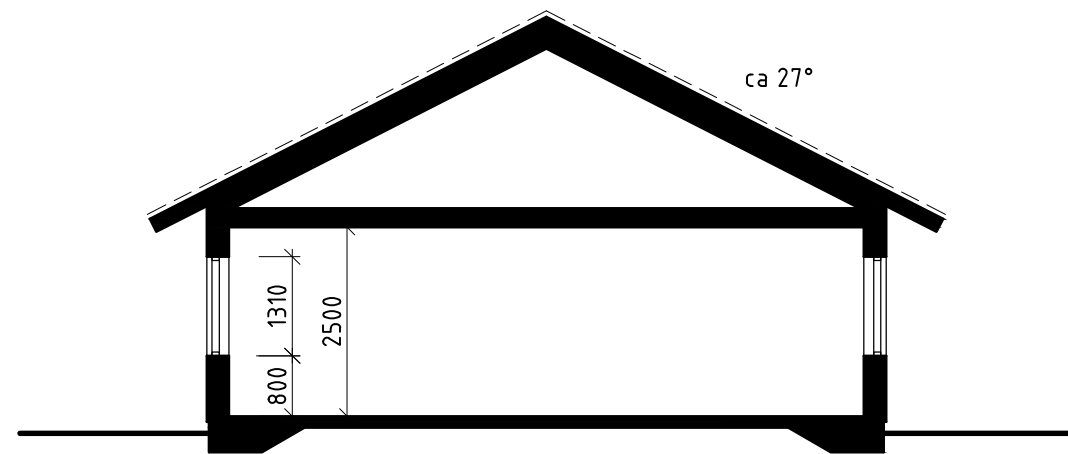
PRINCIPSEKTION
