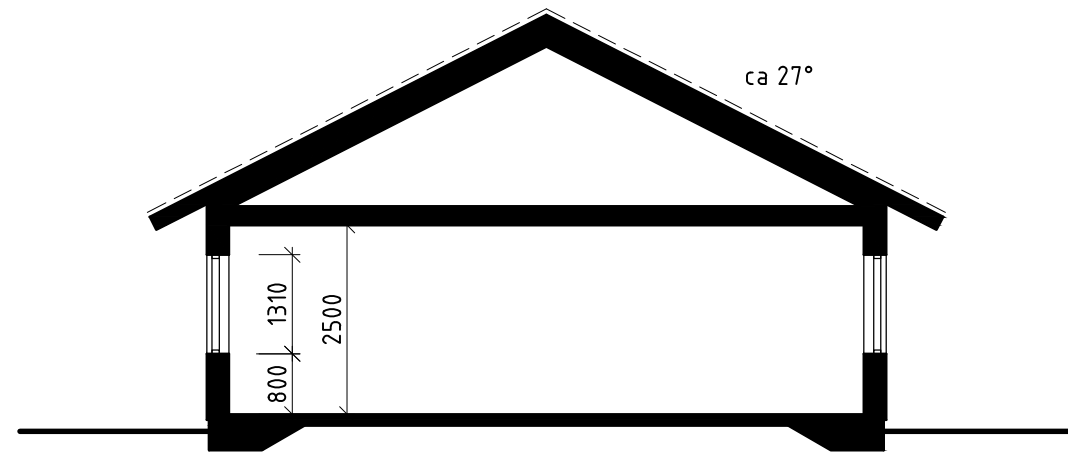
PRINCIPSEKTION
