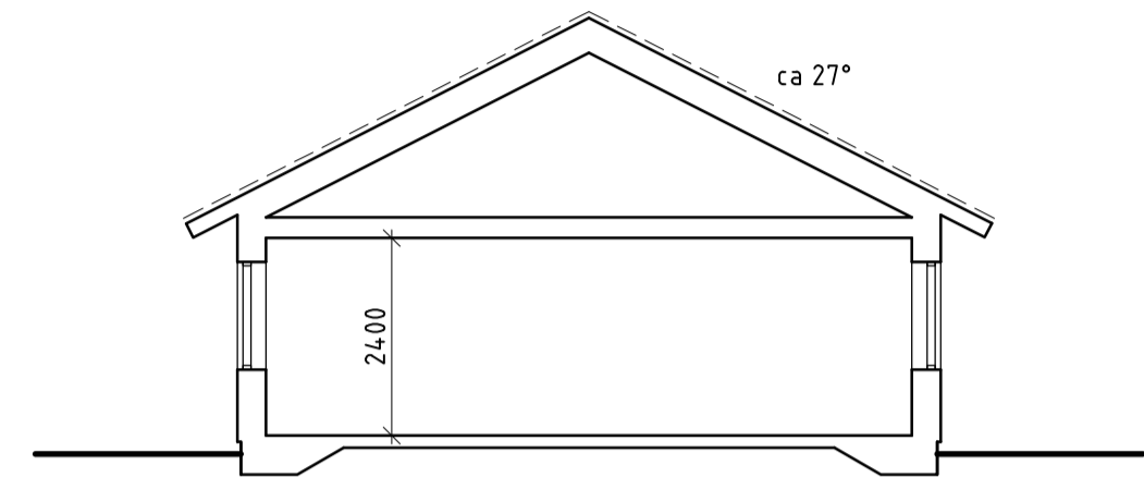
SEKTION A - A
