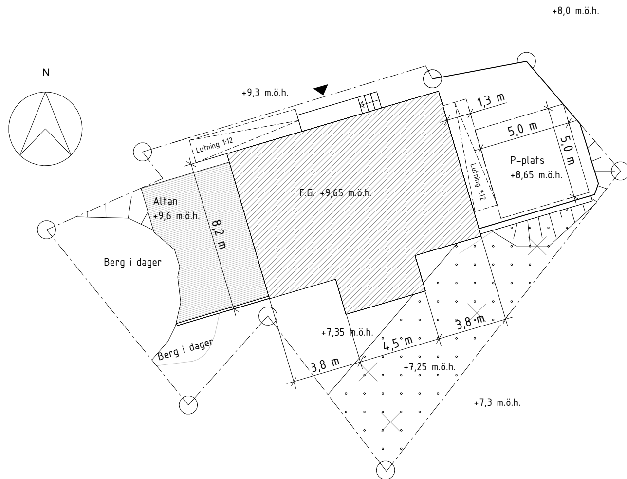
MARKPLANERINGSRITNING
