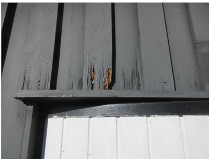
Rötskadad fasadpanel
