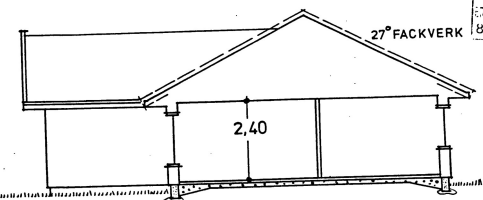
SEKTION
