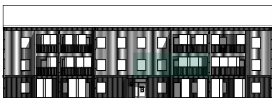
FASAD MOT SYDVÄST
