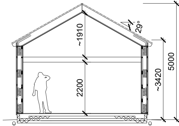
FASAD MOT SYDÖST
