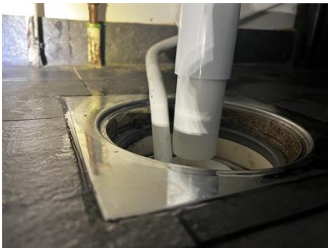
Rör genomföringar placerade i golv-/väggvinkel i tvättstugan.
