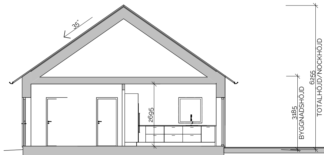
SEKTION A-A
