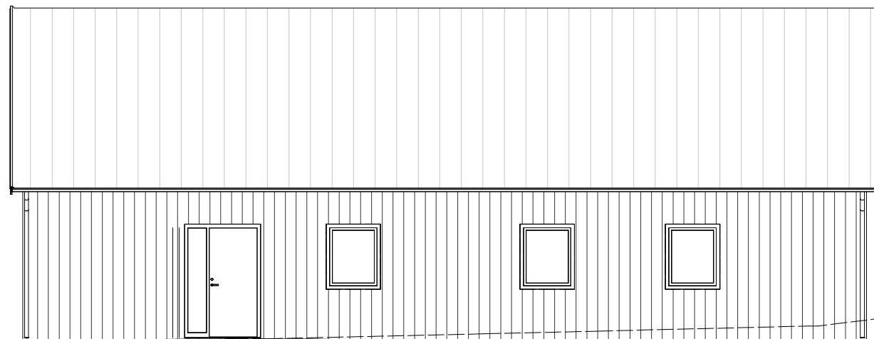
FASAD MOT NORDÖST
