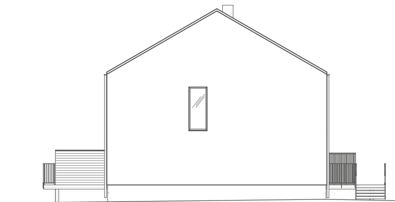
VÄNSTER GAVEL
