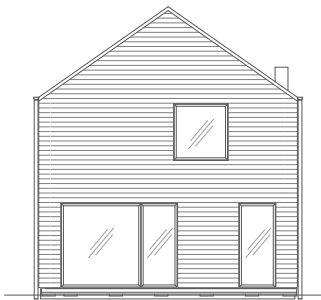
FASAD TRÄDGÅRDSSIDA
