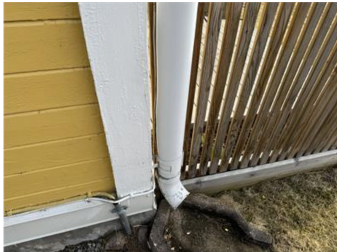
Frostsprängda stuprör med fals mot vägg.
