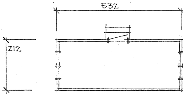
PLAN / ARBETSBOD /
