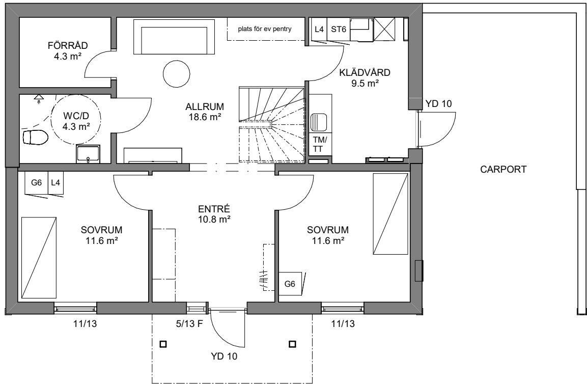
ENTRÉPLAN
