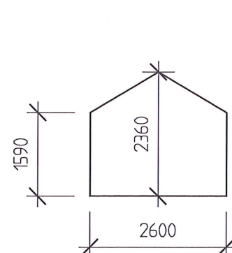
SEKTION B-B
