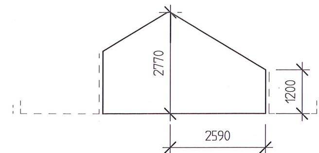
SEKTION D-D
