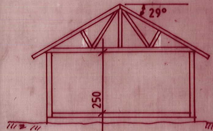
SEKTION A-A
