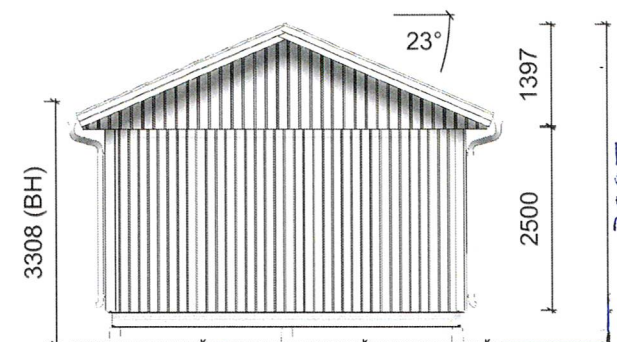
FASAD MOT.....Grannar / SV
