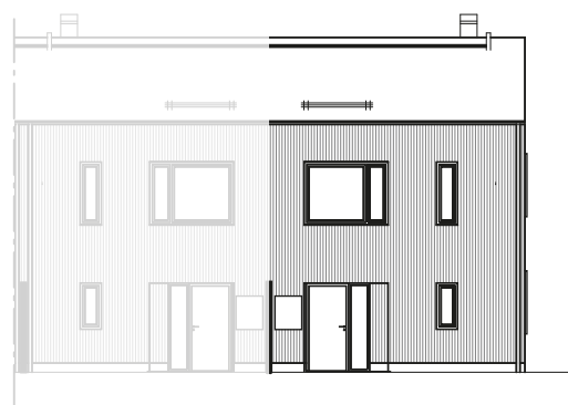
Fasad mot norr del 2
