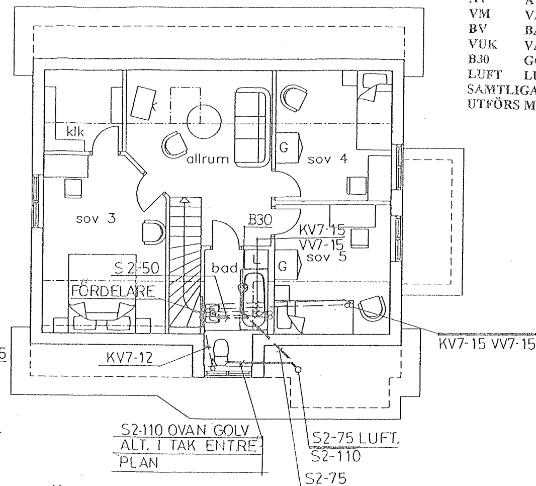
Överplan, 62,0 kvm BRA
