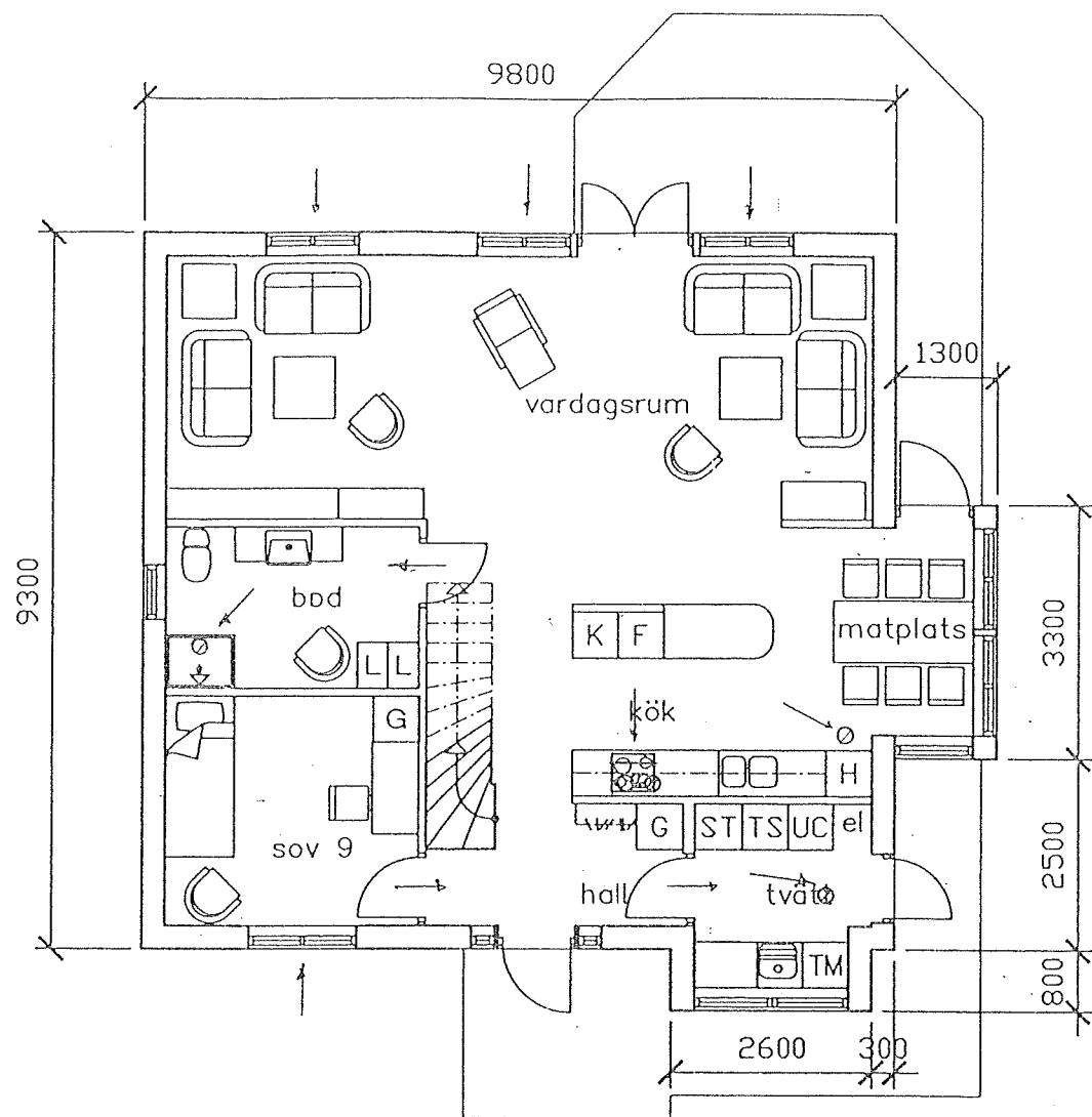
Entréplan, 85,1kvm BRA
