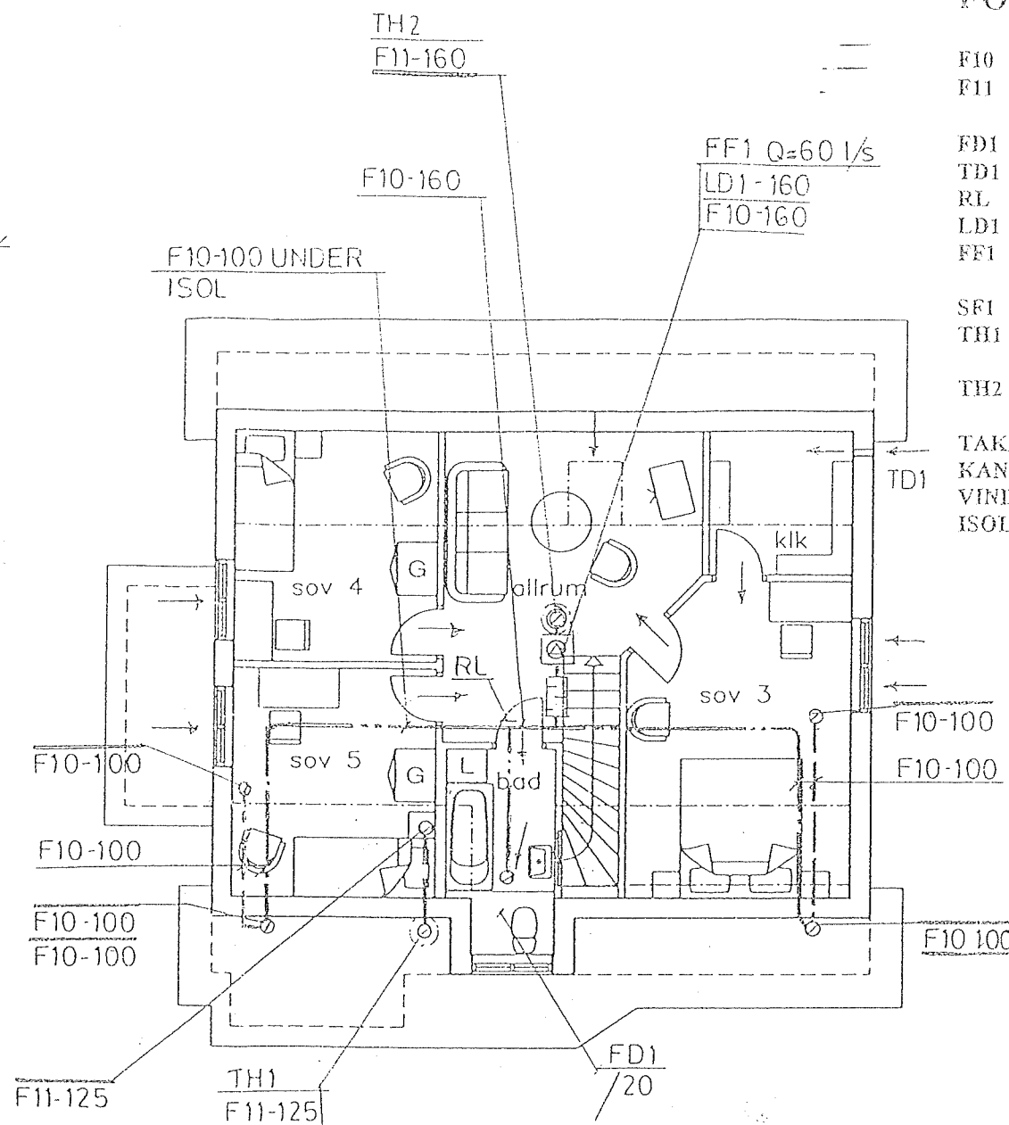
Överplan, 62,0 kvm BRA
