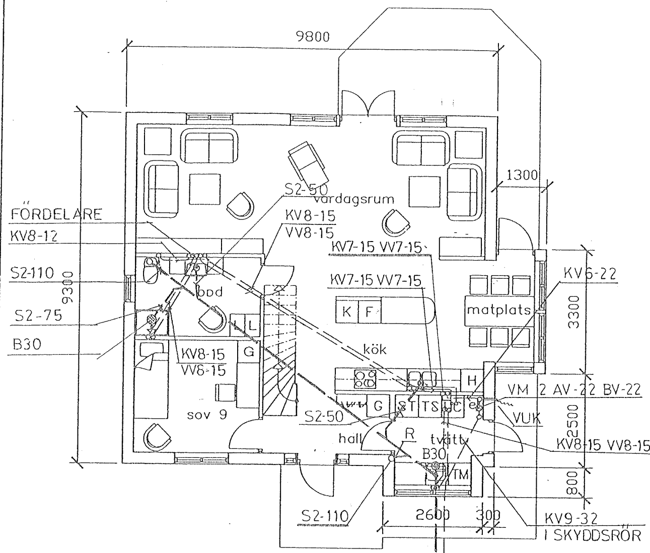
Entréplan, 85,1kvm BRA
