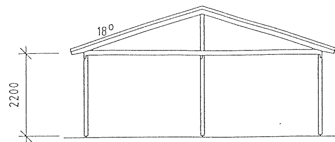
Sektion
