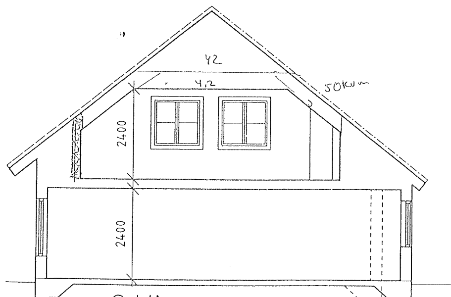
Sektion
