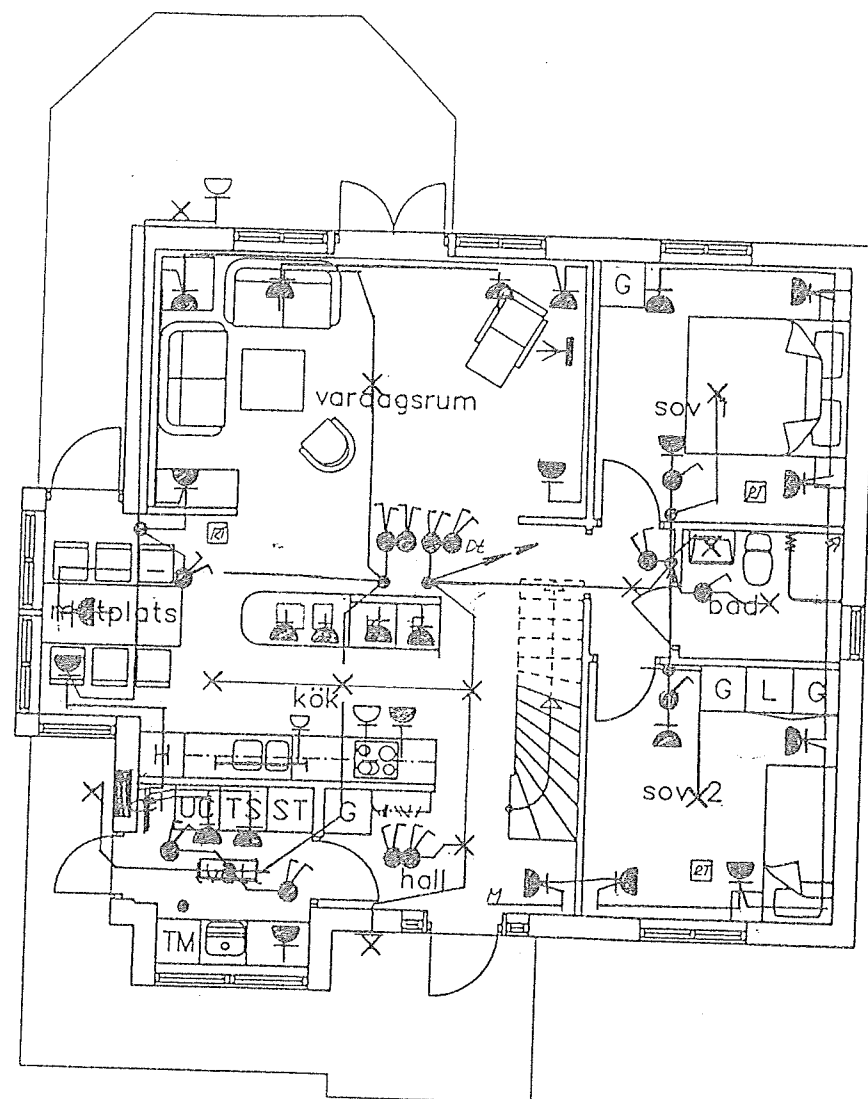
Entréplan, 85,1 kvm BRA
