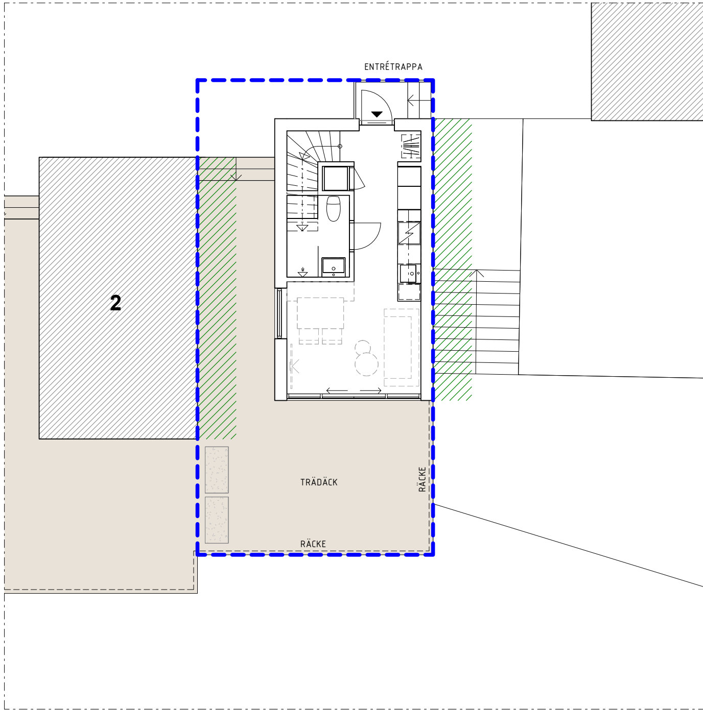
PLANRITNING FISKESTUGA 1
